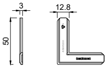
4585130 Kunststoff Eckverbinder Stärke 3,0 mm
