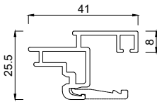
2133841 Flügelprofil 41 mm VB
