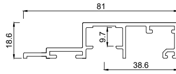
2141081 Einspannprofil 81 mm SL
