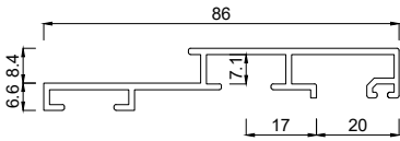
2451186 Einspannrahmenprofil 86 mm FVNG
