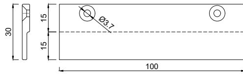
1152430 Glasauflage 4x30/15 mm FB12
