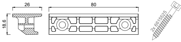
6921026 Glasauflage 26 mm mit 2 Schrauben 5,5x25
