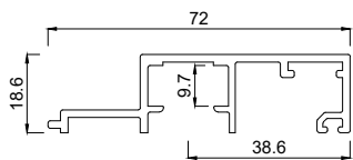
2141072 Rahmenprofil 72 mm SL
