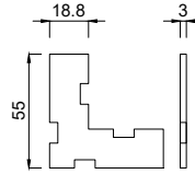
4485030 Aluminium Eckverbinder Stärke 3,0 mm
