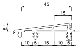
3351450 Mitteldichtung SE (Anschlag 15 mm, Nut 10+5)
