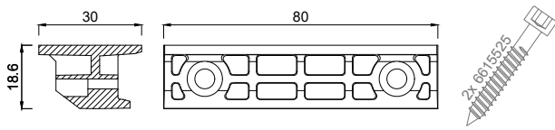
6921030 Glasauflage 30 mm mit 2 Schrauben 5,5x25
