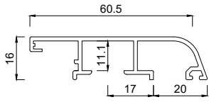
2161066 Rahmenprofil 66 mm gerundet
