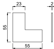
4485232 Aluminium Aussteifungswinkel 23 mm, Stärke 2 mm
