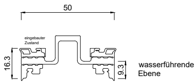
3322200 Pfostendichtung 50 mm innen
