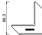
4531970 Aussteifungswinkel Kunststoff
