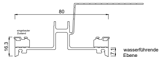
3384100 Riegeldichtung 80 mm (Fußpunkt) innen mit Fahne
