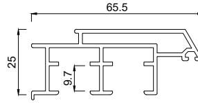
2153165 Flügelprofil 65,5 mm FB12
