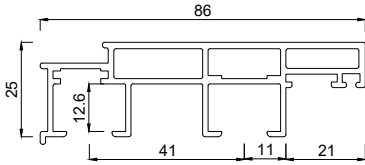
2153786 Flügelprofil 86 mm FB12NG
