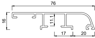
2161076 Rahmenprofil 76 mm gerundet
