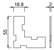
4485020 Aluminium Eckverbinder Stärke 2,0 mm
