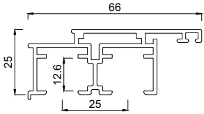
2153666 Flügelprofil 66 mm FB5
