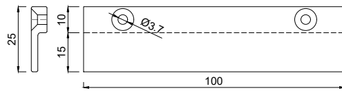
1152625 Glasauflage 6x25/15 mm FB12
