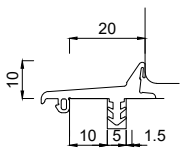
3351200 Mitteldichtung (Anschlag 20 mm, Nut 10+5)
