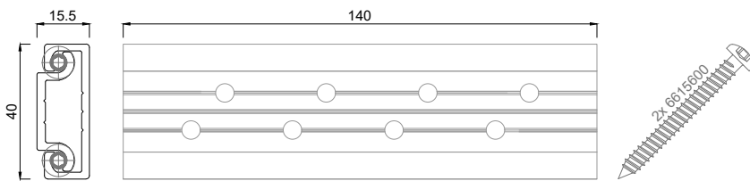
6925140 Pfosten-Riegel Verbinder 140 mm, mit 2 Schrauben 5,5x50
