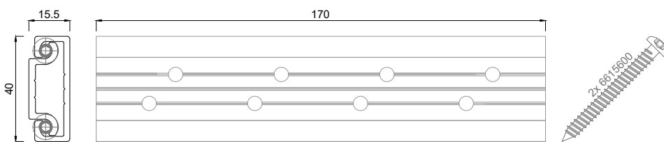
6925170 Pfosten-Riegel Verbinder 170 mm, mit 2 Schrauben 5,5x50 und 2 Stahlstiften
