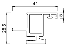
2453941 Flügelprofil 41 mm VB FVNG
