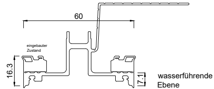
3364100 Riegeldichtung 60 mm (Fußpunkt) innen mit Fahne
