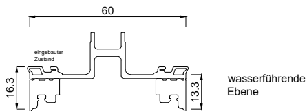
3364300 Riegeldichtung 60 mm innen
