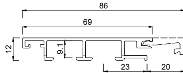
2352069 Rahmenprofil 69 mm FO mit Entwässerung
