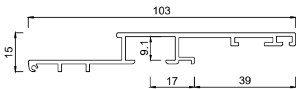
2151103 Einspannrahmenprofil 103 mm IN
