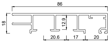
2451886 Rahmenprofil 86 mm FVNG RA
