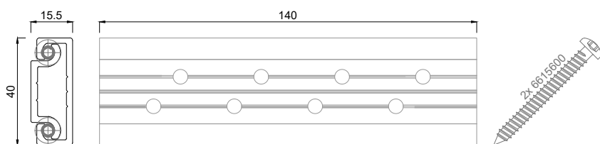
6925140 Pfosten-Riegel Verbinder 140 mm, mit 2 Schrauben 5,5x50
