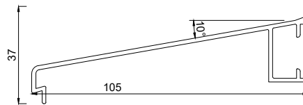
2159105 Abschlussprofil 105 mm
