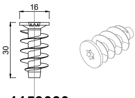
1159030 Schraubhülse SE 16 x 30 mm
