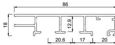
2452886 Rahmenprofil 86 mm FVNG RA mit Entwässerung
