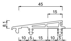
3351450 Mitteldichtung SE (Anschlag 15 mm, Nut 10+5)
