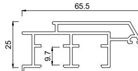
2153165 Flügelprofil 65,5 mm FB12
