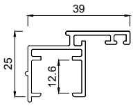
2153939 Flügelprofil 41 mm FB5
