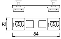
4453084 Schraubverbinder
