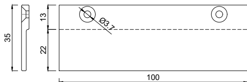
1156435 Glasauflage 4x35/22 mm FB5
