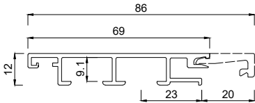
2351069 Rahmenprofil 69 mm FO
