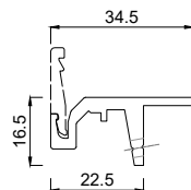
2153016 Flügelprofil 15,0 mm IN
