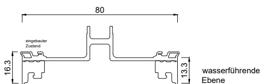
3384300 Riegeldichtung 80 mm innen
