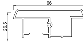
2158066 Stulpprofil 66 mm FV
