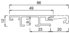
2351049 Rahmenprofil 49 mm FO
