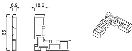
4484069 Druckguss Eckverbinder Stärke 6,9 mm
