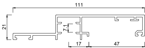
2141111 Einspannrahmenprofil 111 mm INRA
