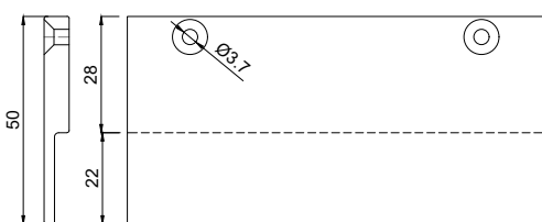
1156650 Glasauflage 6x50/22 mm FB5
