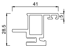
2453941 Flügelprofil 41 mm VB FVNG
