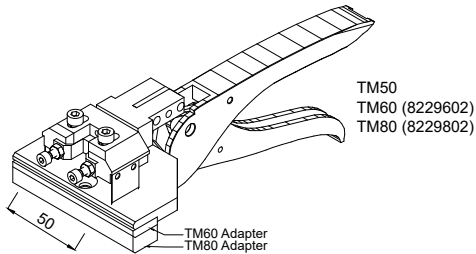
8222502 TM-Dichtungsschere Pfostendichtung
