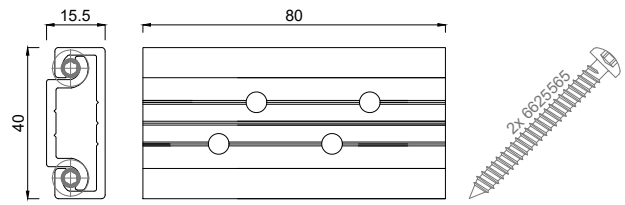
6925080 Pfosten-Riegel Verbinder 80 mm, mit 2 Schrauben 5,5 x 65
