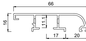
2162066 Rahmenprofil 66 mm gerundet mit Entwässerung
