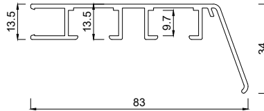
2413483 Flügelprofil 83/34 mm IV
