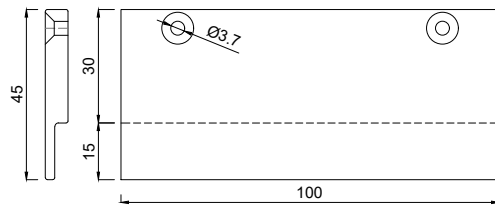
1152645 Glasauflage 6x45/15 mm FB12
