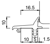
3351165 Mitteldichtung (Anschlag 16,5 mm, Nut 10+5)
