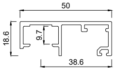
2141050 Rahmenprofil 50 mm SL
