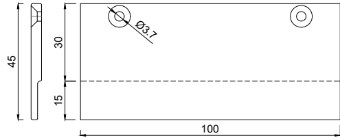
1152445 Glasauflage 4x45/15 mm FB12
