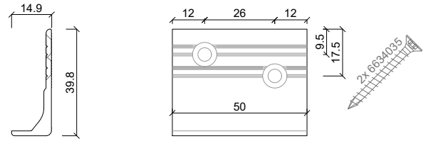
4451540 Aluminiumhaltewinkel (absturzsichernd) FV/FVNG
