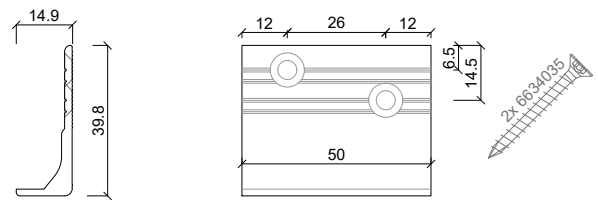
4431540 Aluminiumhaltewinkel (absturzsichernd) FB
