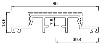
2148080 Stulpprofil 80 mm SL (Verwendung mit 2117012)
