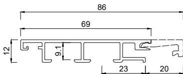
2351069 Rahmenprofil 69 mm FO
