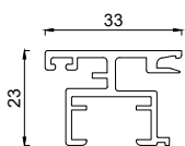
2351033 Rahmenprofil 25 mm FO
