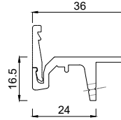
2153416 Flügelprofil 16,5 mm IN
