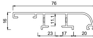
2162076 Rahmenprofil 76 mm gerundet mit Entwässerung
