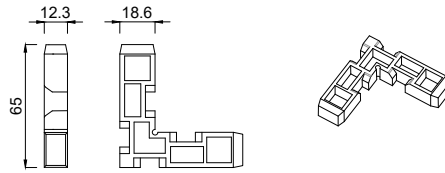
4484123 Druckguss Eckverbinder Stärke 12,3 mm
