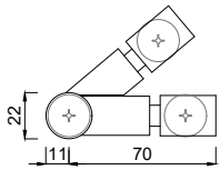
4482040 Schraubverbinder Eckwinkel verstellbar
