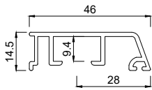
2153046 Flügelprofil 46 mm FV
