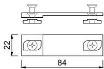
4455084 Schraubverbinder
