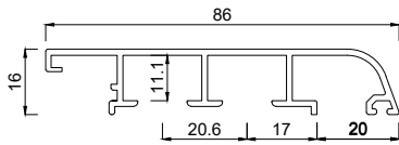
2161086 Rahmenprofil 86 mm gerundet
