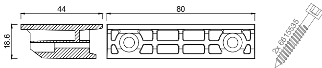
6921044 Glasauflage 44 mm mit 2 Schrauben 5,5x35
