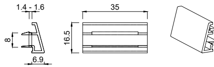
1481000 Entwässerungskappe Metall
