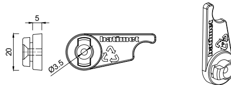
1183005 Drehhalter 5 mm (grün)
