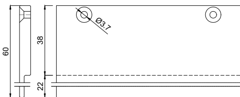
1156660 Glasauflage 6x60/22 mm FB5
