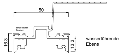
3324400 Riegeldichtung 50 mm innen mit Fahne
