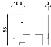
4485030 Aluminium Eckverbinder Stärke 3,0 mm
