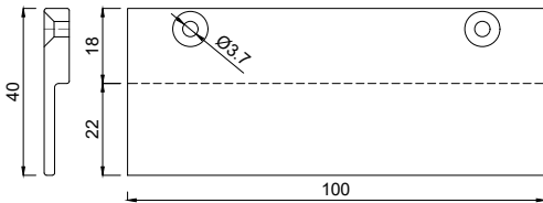
1156640 Glasauflage 6x40/22 mm FB5
