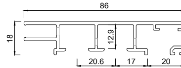
2452886 Rahmenprofil 86 mm FVNG RA mit Entwässerung
