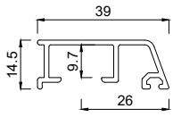
2153039 Flügelprofil 39 mm FV
