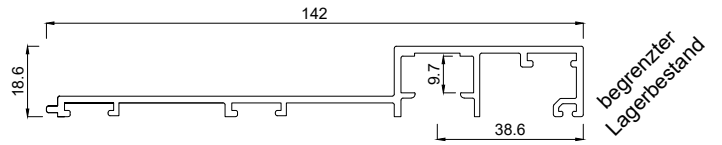
2141142 Rahmenprofil 142 mm SL
