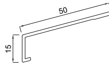
2379515 Wetterschenkel 50 x 15 mm
