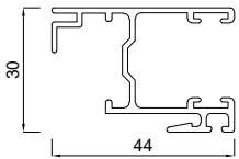
2184344 Rollladenführungsprofil 44 x 30 mm
