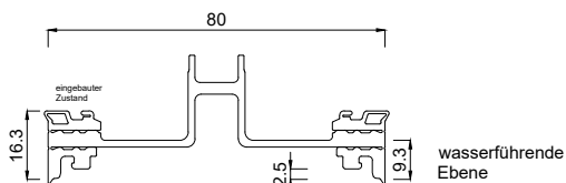
3382200 Pfostendichtung 80 mm innen
