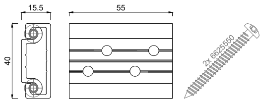
6925055 Pfosten-Riegel Verbinder 55 mm, mit 2 Schrauben 5,5x50
