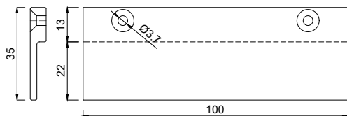
1156635 Glasauflage 6x35/22 mm FB5
