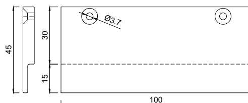
1152645 Glasauflage 6x45/15 mm FB12
