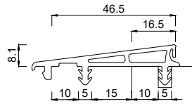
3351465 Mitteldichtung SE (Anschlag 16,5 mm, Nut 10+5)
