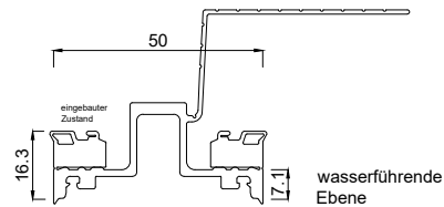
3324100 Riegeldichtung 50 mm (Fußpunkt) innen mit Fahne
