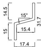
2189015 Z-Kopplungsprofil
