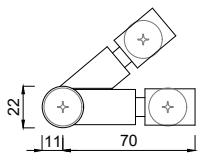
4482040 Schraubverbinder Eckwinkel verstellbar
