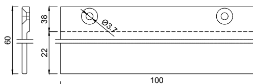
1156460 Glasauflage 4x60/22 mm FB5
