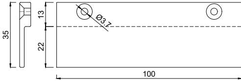
1156635 Glasauflage 6x35/22 mm FB5
