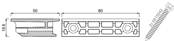
6921050 Glasauflage 50 mm mit 2 Schrauben 5,5x42
