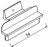
1358054 Endkappen für Stulpprofil 54 mm FV
