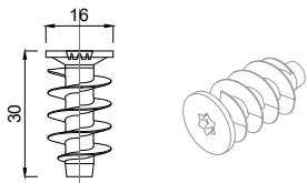
1159030 Schraubhülse SE 16 x 30 mm
