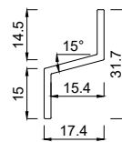
2189015 Z-Kopplungsprofil
