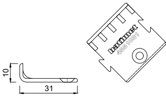
4451031 Haltewinkel für Festverglasung 31x10 mm IN
