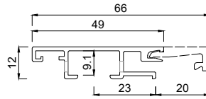
2352049 Rahmenprofil 49 mm FO mit Entwässerung
