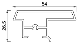
2158054 Stulpprofil 54 mm FV
