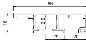
2452866 Rahmenprofil 66 mm FVNG RA mit Entwässerung
