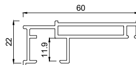
2153460 Blechapplikationsprofil 60 mm FB
