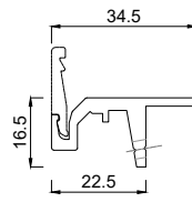
2153016 Flügelprofil 15,0 mm IN
