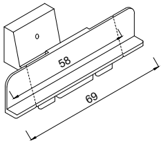
1338600 Endkappen für Stulpprofil 69 / 58 mm FB
