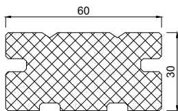
3952060 SE-Pad 30 x 60 mm
