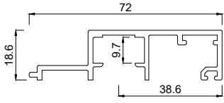
2141072 Rahmenprofil 72 mm SL
