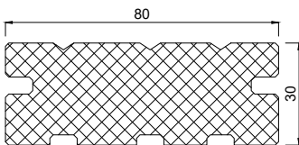
3952080 SE-Pad 30 x 80 mm
