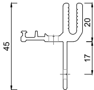
2121632 Grundprofil 32 mm für Dehnpfosten TM60, Schraubkanal
