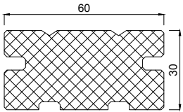
3952060 SE-Pad 30 x 60 mm
