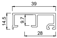
2453039 Flügelprofil 39 mm FVNG
