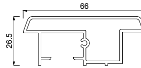
2158066 Stulpprofil 66 mm FV
