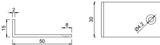
4451350 Haltewinkel für Festverglasung 50x15 mm SE
