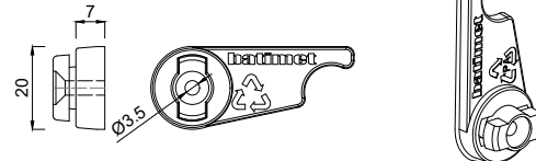
1183007 Drehhalter 7 mm (blau)
