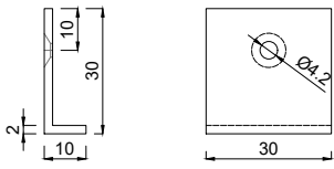
4431030 Haltewinkel für Festverglasung 30x10 mm FO
