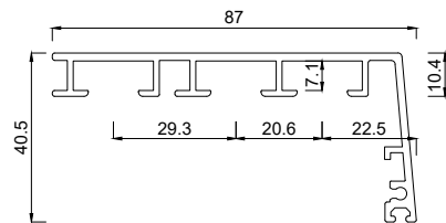
2411087 Rahmenprofil 87 mm IV
