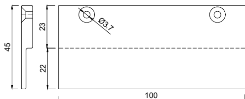
1156645 Glasauflage 6x45/22 mm FB5
