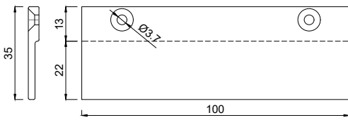
1156435 Glasauflage 4x35/22 mm FB5
