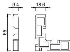
4484094 Druckguss Eckverbinder Stärke 9,4 mm
