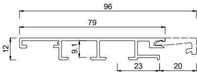
2351079 Rahmenprofil 79 mm FO
