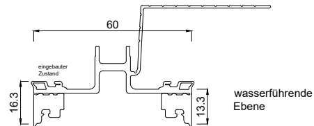
3364400 Riegeldichtung 60 mm innen mit Fahne
