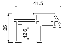
2153541 Flügelprofil 41,5 mm FB12
