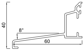
2159640 Wetterschenkelprofil 60 x 40 mm
