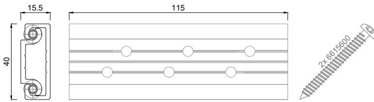
6925115 Pfosten-Riegel Verbinder 115 mm, mit 2 Schrauben 5,5x50
