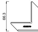
4531970 Aussteifungswinkel Kunststoff
