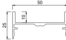
2117025 Abdeckprofil 50 mm, 25 mm, U-Profil
