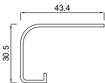
2184430 Abrollprofil für Rollladen 43,4 x 30,5 mm
