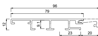
2352079 Rahmenprofil 79 mm FO mit Entwässerung
