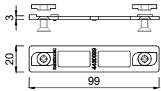
4430099 Schraubverbinder
