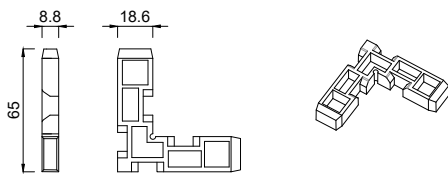
4484088 Druckguss Eckverbinder Stärke 8,8 mm
