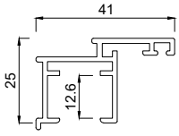
2153941 Flügelprofil 41 mm FB5
