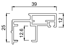
2133739 Flügelprofil 39 mm FB12NG
