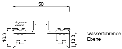
3324300 Riegeldichtung 50 mm innen
