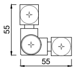
4482090 Schraubverbinder Eckwinkel 90°
