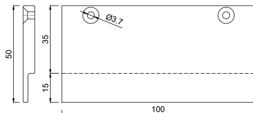
1152650 Glasauflage 6x50/15 mm FB12
