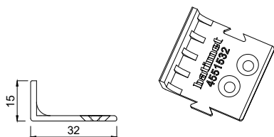
4551532 Haltewinkel für Festverglasung 32x15 mm FB/FV/FVNG
