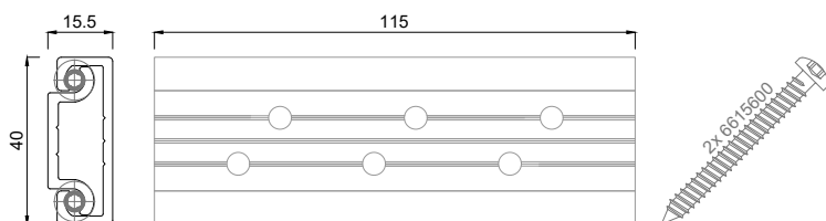
6925115 Pfosten-Riegel Verbinder 115 mm, mit 2 Schrauben 5,5x50
