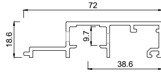
2142072 Rahmenprofil 72 mm SL mit Entwässerung
