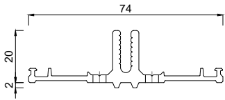
2121080 Grundprofil 80 mm
