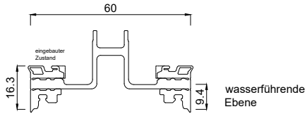
3362200 Pfostendichtung 60 mm innen
