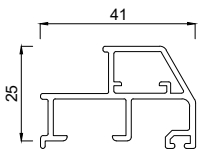
2453541 Flügelprofil 41 mm FBNG
