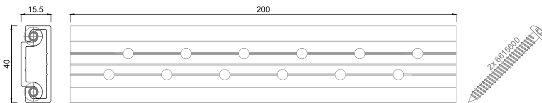
6925200 Pfosten-Riegel Verbinder 200 mm, mit 2 Schrauben 5,5x50 und 2 Stahlstiften
