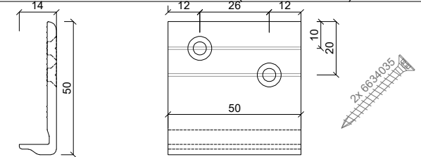
4451550 Aluminiumhaltewinkel (absturzsichernd) FO
