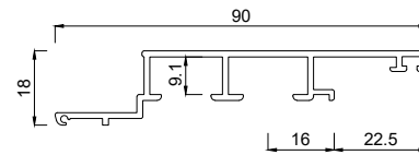
2131190 Einspannrahmenprofil 90 mm FB
