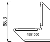
4551550 Aussteifungswinkel Kunststoff
