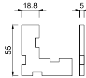
4485050 Aluminium Eckverbinder Stärke 5,0 mm
