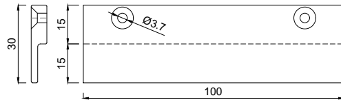
1152630 Glasauflage 6x30/15 mm FB12
