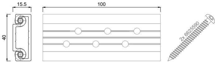
6925100 Pfosten-Riegel Verbinder 100 mm, mit 2 Schrauben 5,5x50
