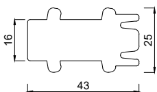
3724454 SE-SPACER Glasstärke 44 - 54 mm
