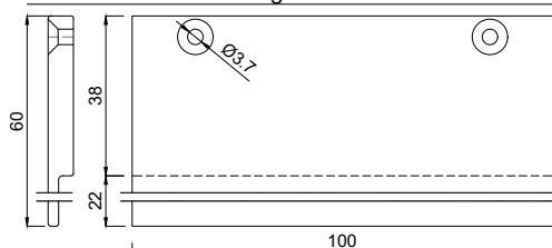
1156660 Glasauflage 6x60/22 mm FB5
