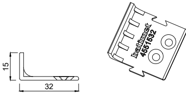
4451532 Haltewinkel für Festverglasung 32x15 mm FB/FV/FVNG
