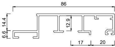
2451986 Einspannrahmenprofil 86 mm FVNG RA
