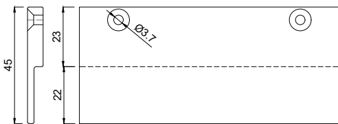
1156645 Glasauflage 6x45/22 mm FB5
