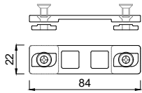
4453084 Schraubverbinder
