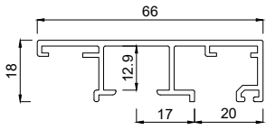
2451866 Rahmenprofil 66 mm FVNG RA
