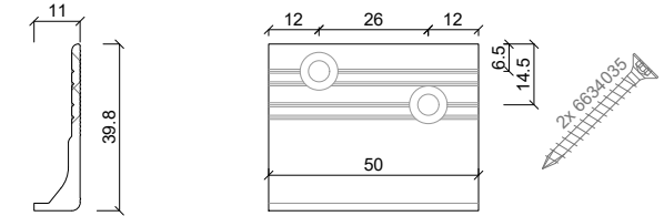
4451140 Aluminiumhaltewinkel (absturzsichernd) IN
