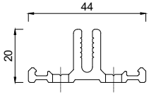
2122000 Grundprofil 50 mm ohne Führung
