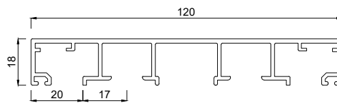
2457120 Setzholzprofil 120 mm FVNG RA
