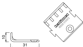
4551031 Haltewinkel für Festverglasung 31x10 mm IN
