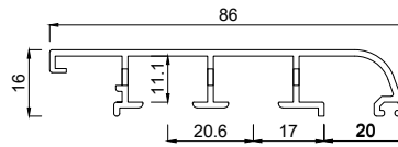
2162086 Rahmenprofil 86 mm gerundet mit Entwässerung
