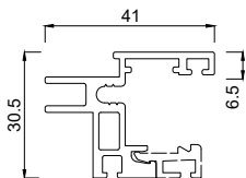
2133941 Flügelprofil 24 mm VB
