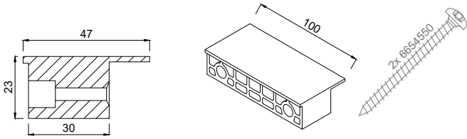
6951030 Glasauflage SE, inkl. 2 Schrauben 4,5x50
