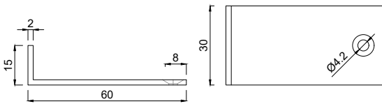
4451360 Haltewinkel für Festverglasung 60x15 mm SE
