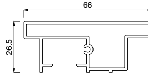
2458066 Stulpprofil 66 mm FVNG
