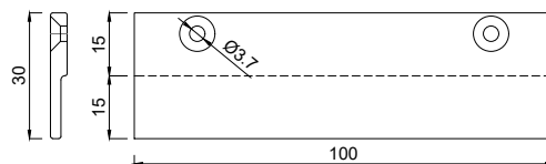
1152430 Glasauflage 4x30/15 mm FB12
