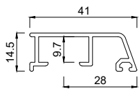
2153041 Flügelprofil 41 mm FV
