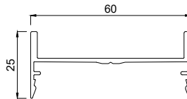
2126025 Abdeckprofil 60 mm, 25 mm U-Profil
