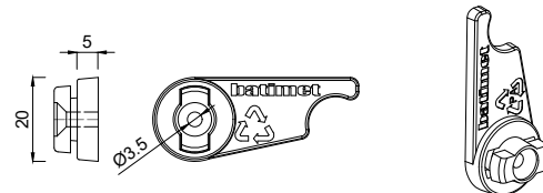
1183005 Drehhalter 5 mm (grün)
