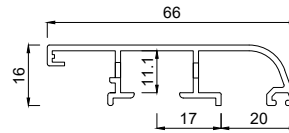
2162066 Rahmenprofil 66 mm gerundet mit Entwässerung
