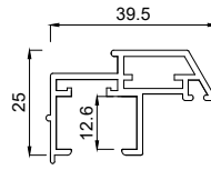
2153539 Flügelprofil 39,5 mm FB12
