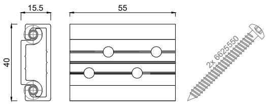
6925055 Pfosten-Riegel Verbinder 55 mm, mit 2 Schrauben 5,5x50
