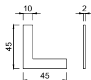
4485102 Aluminium Aussteifungswinkel 10 mm, Stärke 2,0 mm
