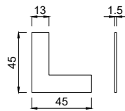
4485131 Aluminium Aussteifungswinkel 13 mm, Stärke 1,5 mm
