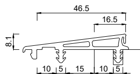
3351465 Mitteldichtung SE (Anschlag 16,5 mm, Nut 10+5)
