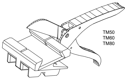
8222501 TM-Dichtungsschere Trennschnitt
