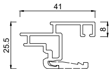
2133841 Flügelprofil 41 mm VB
