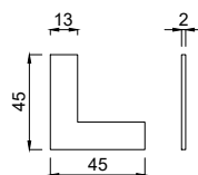
4485132 Aluminium Aussteifungswinkel 13 mm, Stärke 2,0 mm
