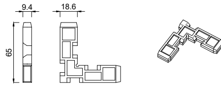
4484094 Druckguss Eckverbinder Stärke 9,4 mm
