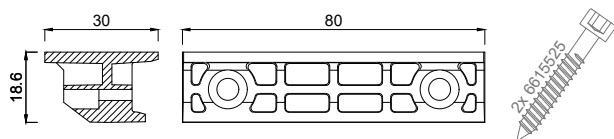
6921030 Glasauflage 30 mm mit 2 Schrauben 5,5x25
