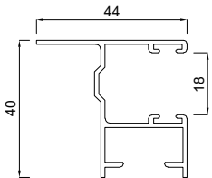
2184044 Rollladenführungsprofil 44 x 40 mm
