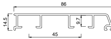
2153086 Flügelprofil 86 mm FV
