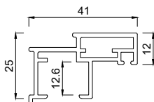
2133741 Flügelprofil 41 mm FB12NG
