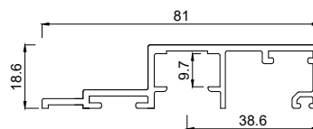
2141081 Einspannrahmenprofil 81 mm SL
