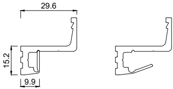
2753031 Flügelprofil SL Kunststoff
