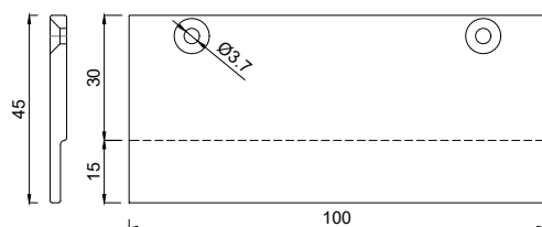
1152445 Glasauflage 4x45/15 mm FB12
