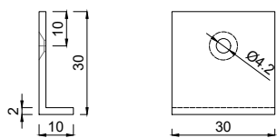
4431030 Haltewinkel für Festverglasung 30x10 mm FO
