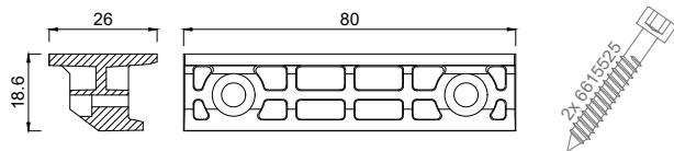
6921026 Glasauflage 26 mm mit 2 Schrauben 5,5x25
