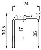
2121624 Grundprofil 24 mm für Dehnpfosten TM60
