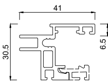
2133941 Flügelprofil 24 mm VB
