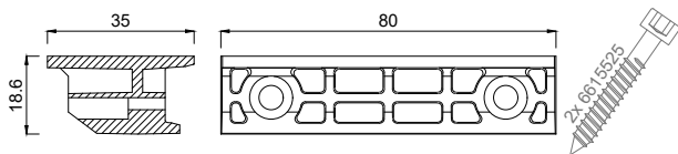
6921035 Glasauflage 35 mm mit 2 Schrauben 5,5x25
