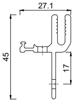
2121027 Grundprofil 27 mm für Dehnpfosten, Schraubkanal
