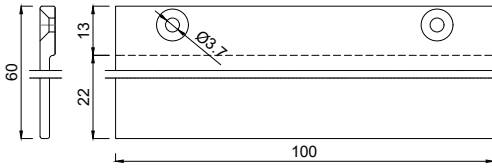
1156460 Glasauflage 4x60/22 mm FB5
