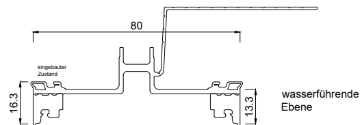
3384400 Riegeldichtung 80 mm innen mit Fahne
