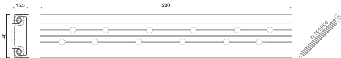
6925230 Pfosten-Riegel Verbinder 230 mm, mit 2 Schrauben 5,5x50 und 2 Stahlstiften
