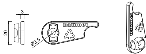
1183003 Drehhalter 3 mm (rot)
