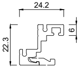
2133924 Flügelprofil 24 mm INVB
