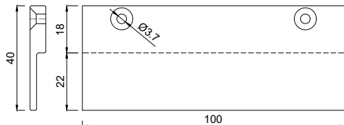
1156640 Glasauflage 6x40/22 mm FB5
