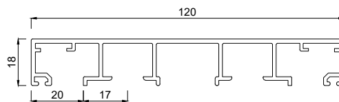
2457120 Setzhholzprofil 120 mm FVNG RA
