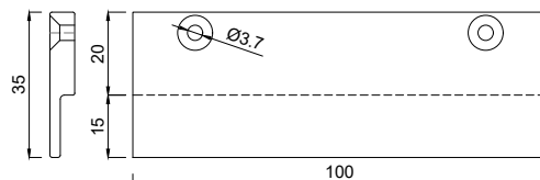
1152635 Glasauflage 6x35/15 mm FB12
