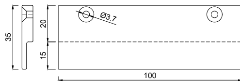
1152635 Glasauflage 6x35/15 mm FB12
