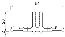
2121060 Grundprofil 60 mm
