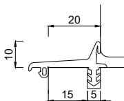
3351215 Mitteldichtung (Anschlag 20 mm, Nut 15+5)
