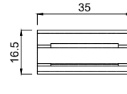
1481000 Entwässerungskappe Metall
