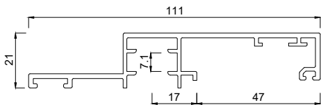
2141111 Einspannrahmenprofil 111 mm INRA
