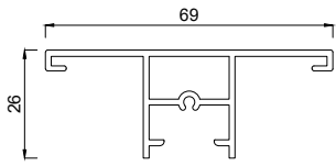
2138069 Stulpprofil 69 mm VB
