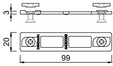
4430099 Schraubverbinder
