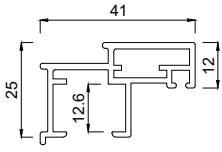
2133741 Flügelprofil 41 mm FB12NG
