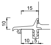
3351100 Mitteldichtung (Anschlag 15 mm)
