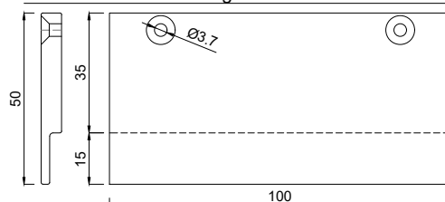
1152650 Glasauflage 6x50/15 mm FB12
