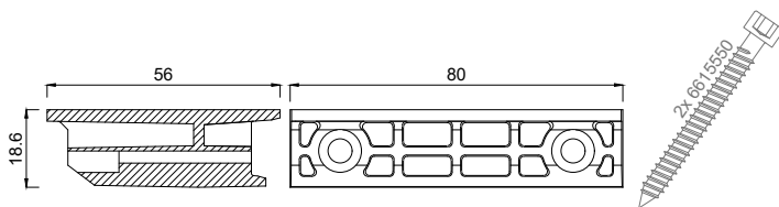
6921056 Glasauflage 56 mm mit 2 Schrauben 5,5x50
