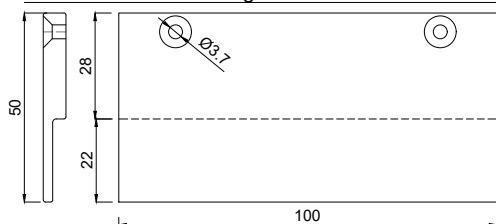
1156650 Glasauflage 6x50/22 mm FB5
