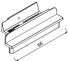
1358466 Endkappen für Stulpprofil 66 mm FVNG
