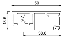
2142050 Rahmenprofil 50 mm SL mit Entwässerung
