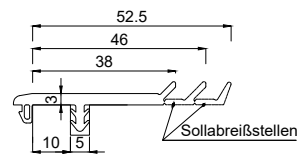
3351960 Festverglasungsdichtung 60 mm
