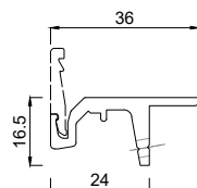
2153416 Flügelprofil 16,5 mm IN
