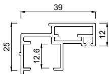
2133739 Flügelprofil 39 mm FB12NG
